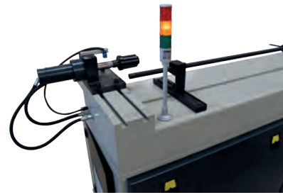
Hydraulischer Dorn
