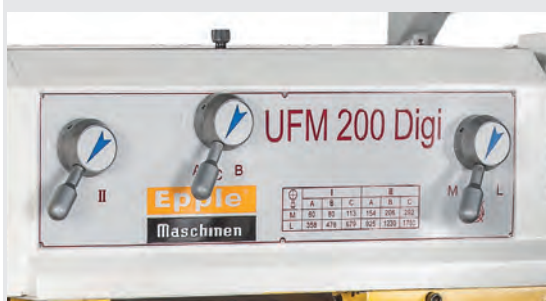
Bedieneinheit zur Einstellung der 12 Spindeldrehzahlen
