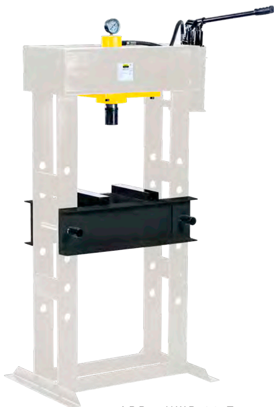
ABB.: HWP 30 T
