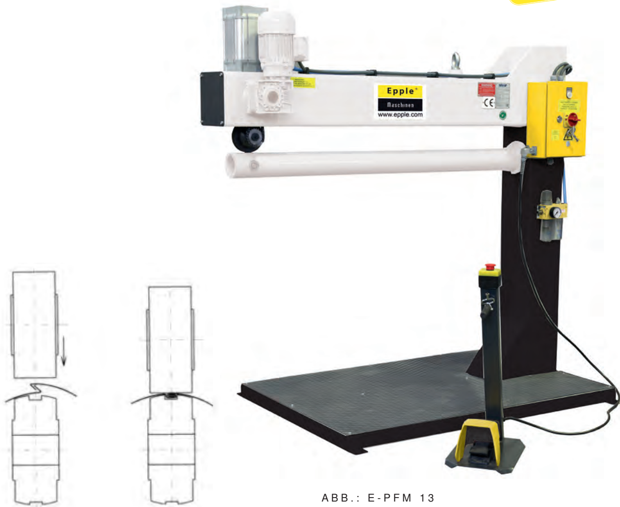
ABB.: SKIZZE DRÜCKPOSITION
