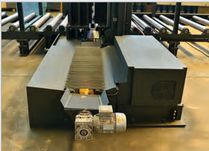
ABB.: SPÄNEFÖRDERER
