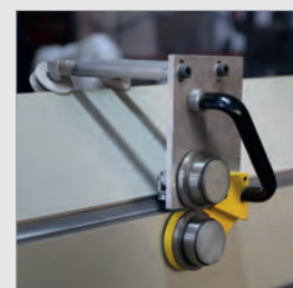
ABB.: SCHNEIDEINHEIT
