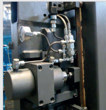
ABB.: HYDRAULISCHE BANDSPANNUNG
