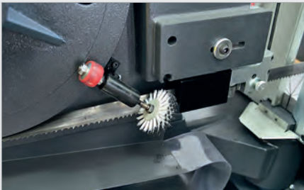
ABB.: SPÄNEBÜRSTE
