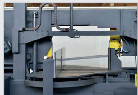
ABB.: HYDRAULISCHE OBERSPANNVORRICHTUNG
