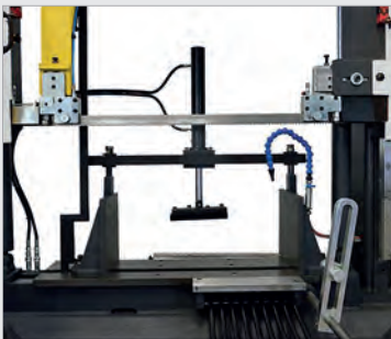
ABB.: HYDRAULISCHE OBERSPANNVORRICHTUNG
