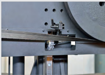
ABB.: MOTORISCHE SPÄNEBÜRSTE
