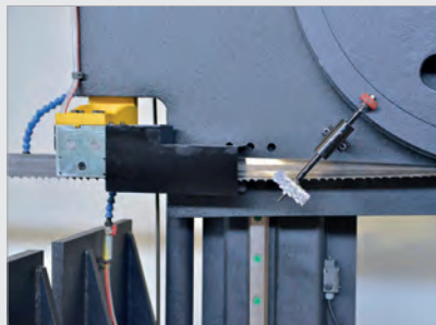
ABB.: SPÄNEBÜRSTE
