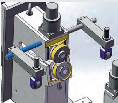
ABB.: E-KS 5 M FLANSCHBEFESTIGUNG
