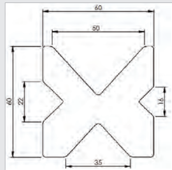
ABB.: 4V UNTERER MATRIZE
