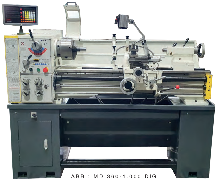
ABB.: MD 360-1.000 DIGI
