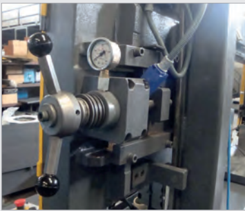
ABB.: HYDRAULISCH-MECHANISCHE BANDSPANNUNG
