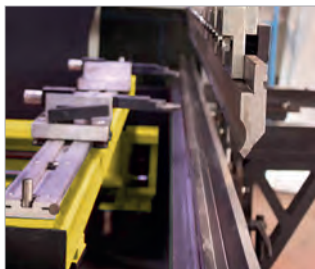
ABB.: PRESSWERKZEUG
