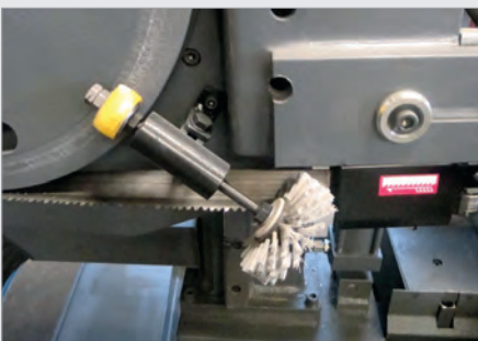
ABB.: SPÄNEBÜRSTE
