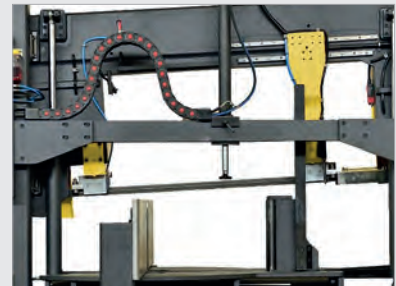
ABB.: HYDRAULISCHE OBERSPANNVORRICHTUNG
