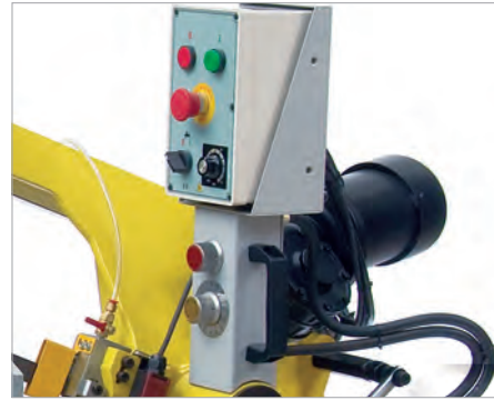
ABB.: ÜBERSICHTLICHES, ERGONOMISCHES BEDIENFELD
